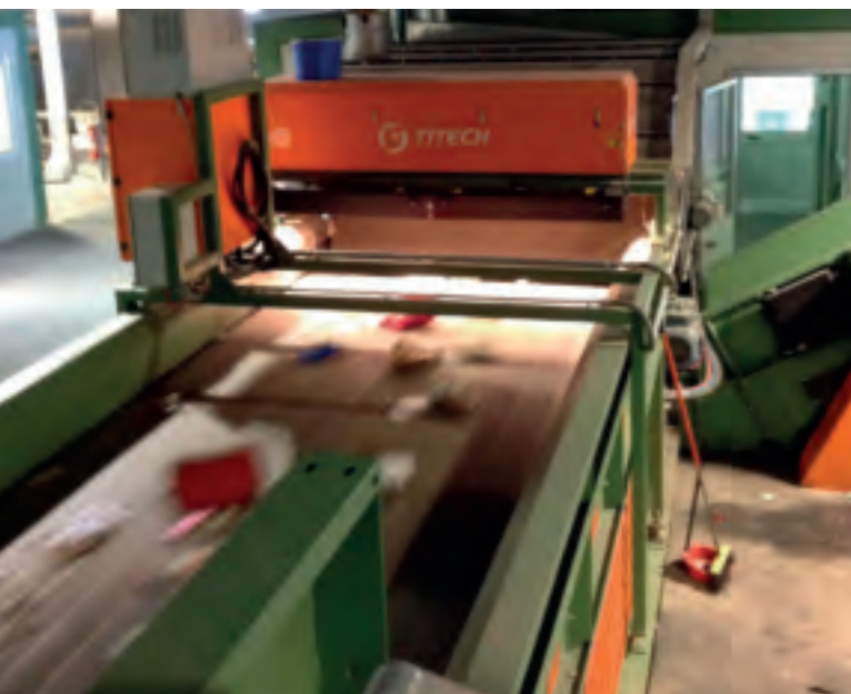
Оптический сепаратор NIR 2000 - NIR 2000 optical separator
